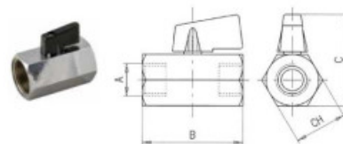
6065 MINI BALL VALVE FEMALE G ISO 228 - FEMALE G ISO 228 MINI-KUGELHAHN INNENGEW. G ISO 228 - INNENGEW. G ISO 228
