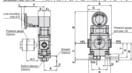
Dimensions AV□2000-A/3000-A/4000-A/5000-A [mm]
